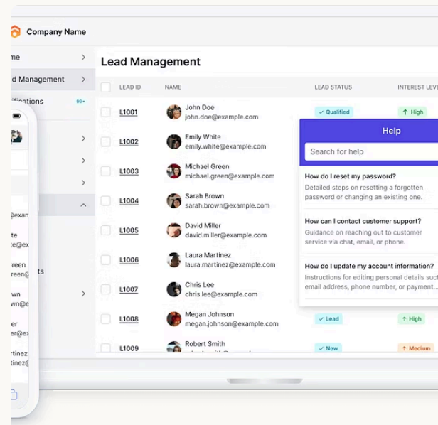
Blazor Server
